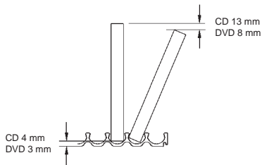
Anwendungsbeispiel mit 5 mm Fachbodenträgern.
